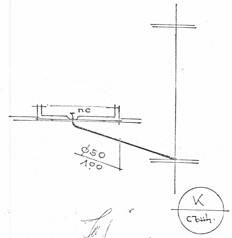
АКСОНОМЕТРИЯ КАНАЛИЗАЦИЯ
