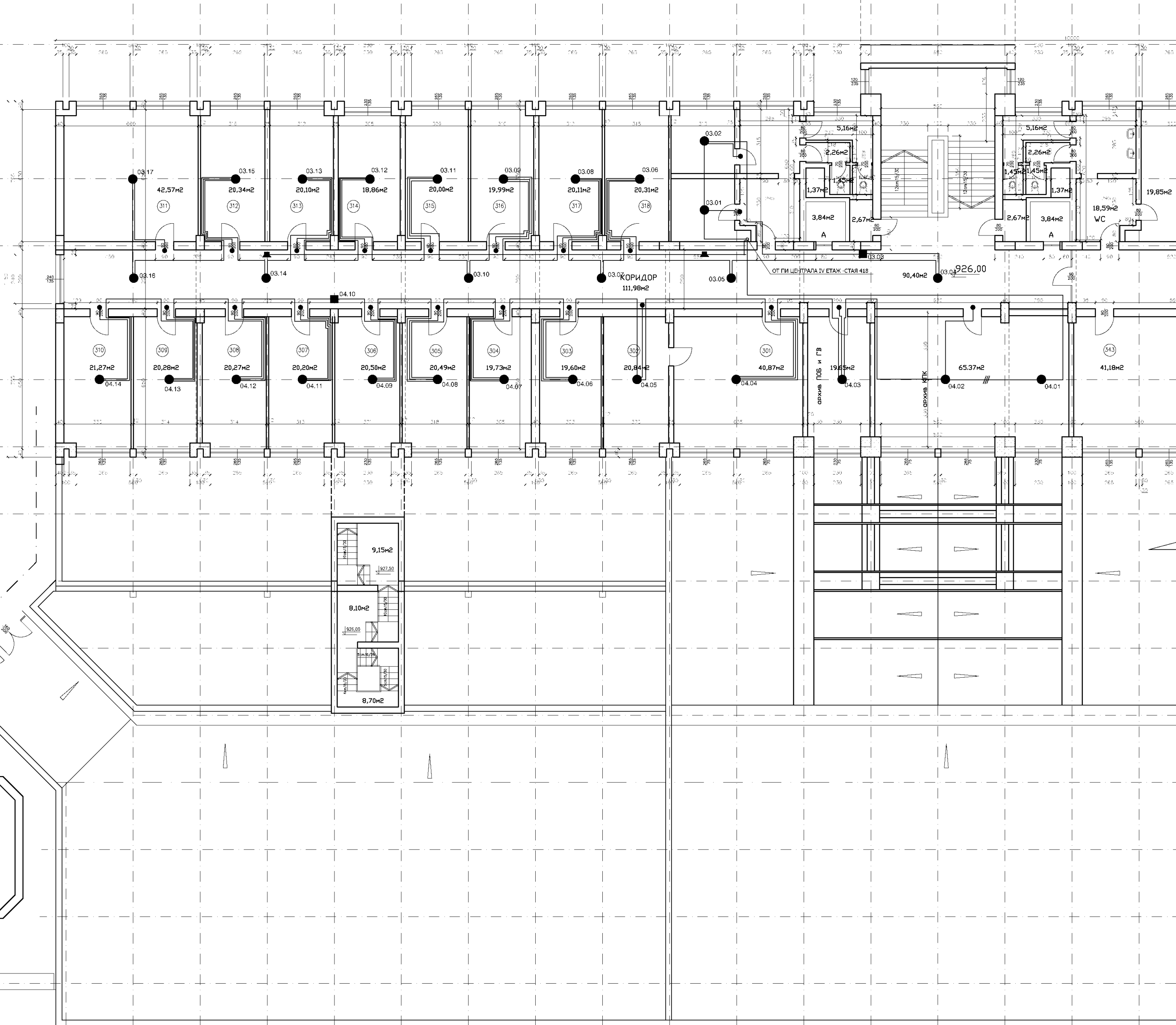
РАЗПРЕДЕЛЕНИЕ ТРЕТИ ЕТАЖ - КОТА - 926,00
